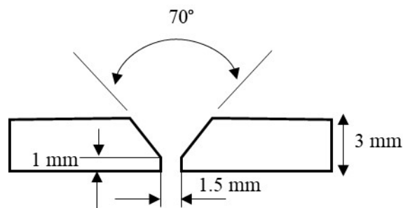
شکل 1- شماتیک طرح اتصال از نمای روبرو.
