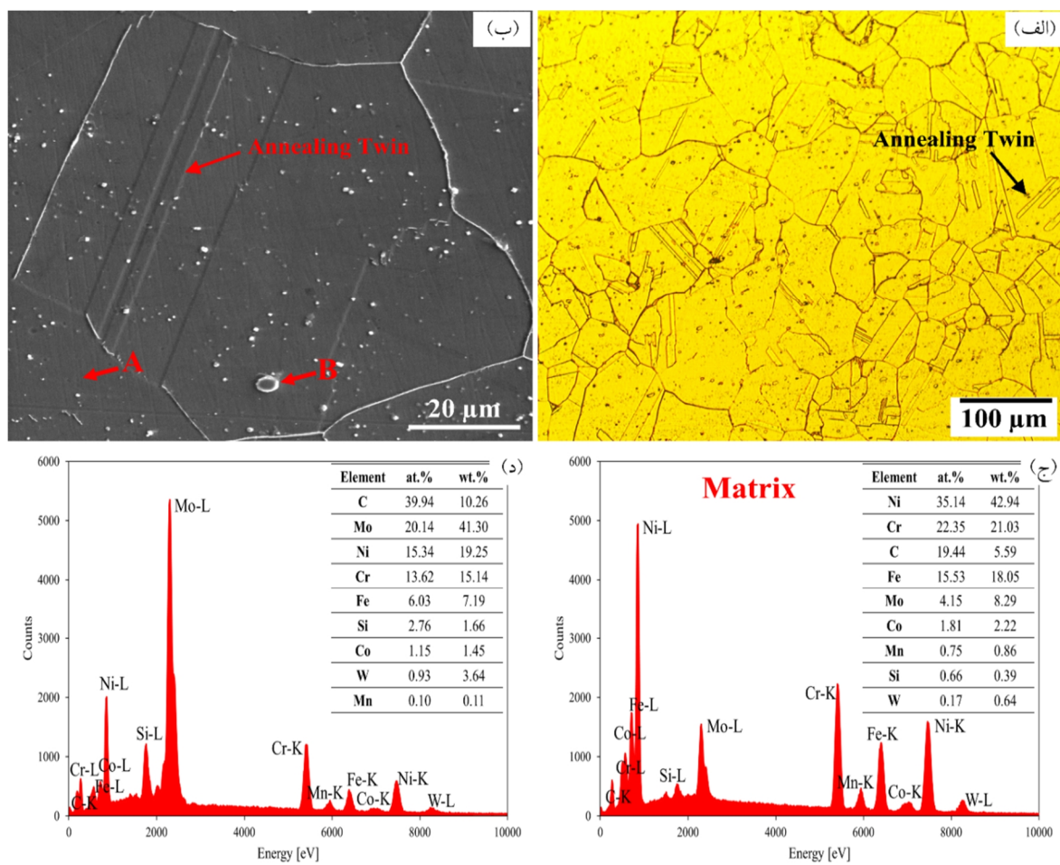
شکل 4- ریزساختار فلزی پایه HX در شرایط آنیل انحلالی
