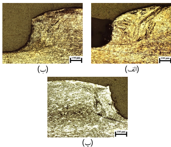
شکل 7- تصویر میکروسکوپی کنار جوش نمونه با مدت زمان تماس 40 ثانیه و سرعت دورانی 1320 (الف)، 1800 (ب) و 2500 (پ)
