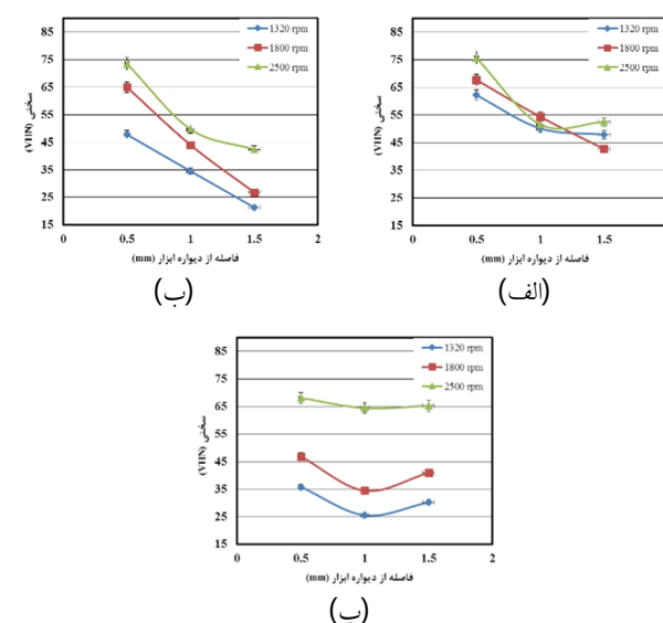
شکل 10- تغییرات سختی نمونه‌ها برحسب فاصله از دیواره ابزار در مدت زمان‌های تماس الف-40 ثانیه، ب-60 ثانیه و ب-80 ثانیه
