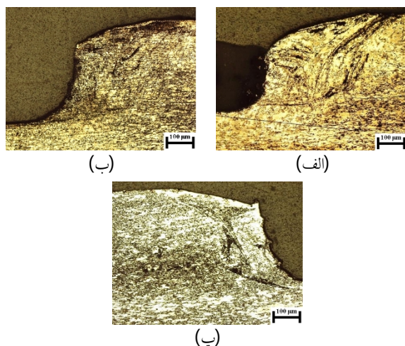
شکل 7- تصویر ماکروسکوپی کنار جوش نمونه با مدت زمان تماس 40 ثانیه و سرعت دورانی 1320 (الف)، 1800 (ب) و 2500 (پ)
