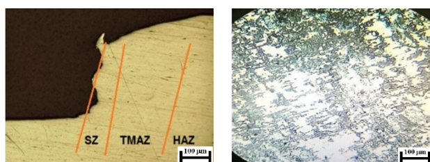
شکل 6- ریزساختار میکروسکوپ نوری از نمونه ماده خام (الف) و مقطع فرایند FSSW بدون عملیات اچ با محدوده تقریبی نواحی سه‌گانه (ب)
