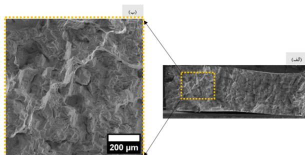
شکل 13- تصویر میکروسکوپ الکترونی نمونه B2 الف - تصویر از مقطع شکست، ب - تصویر با بزرگنمایی بیشتر از قسمت مشخص شده.
