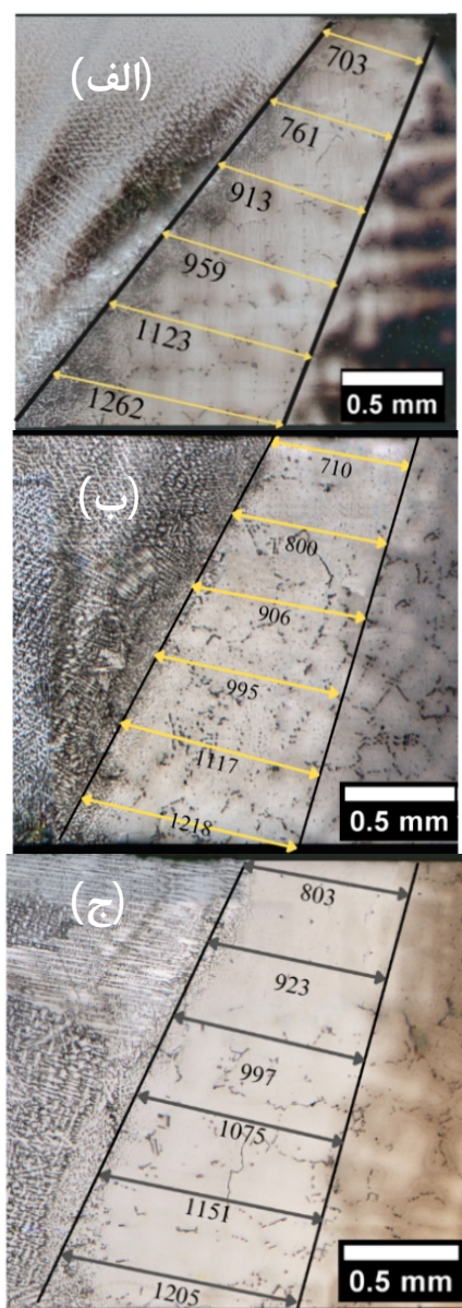
شکل 5- تصویر میکروسکوپ نوری از ناحیه HAZ.
