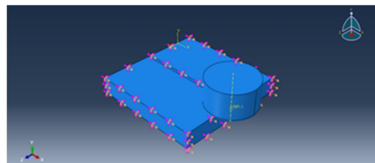
شکل 6- حرکت و بار در جهت ابزار داده شده در نرم افزار آباکوس.
