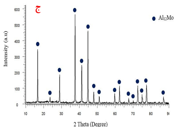
شکل 6- طرح پراش پرتو X از پودر آلیاژسازی مکانیکی شده‌ی مخلوط آلومینیوم و مولیبدن بعد از الف - 40 h و ب - 60 h آلیاژسازی مکانیکی و ج - بعد از عملیات حرارتی نهایی در کوره برای تکمیل واکنش.
