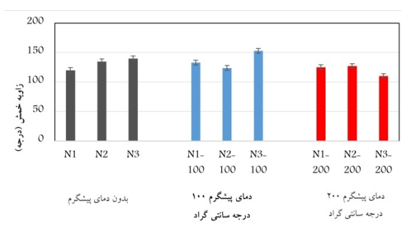
شکل 11- تغییرات زاویه خمش نمونه ها بر حسب تعداد پاس‌ها در شرایط دمایی پیشگرم متفاوت.
