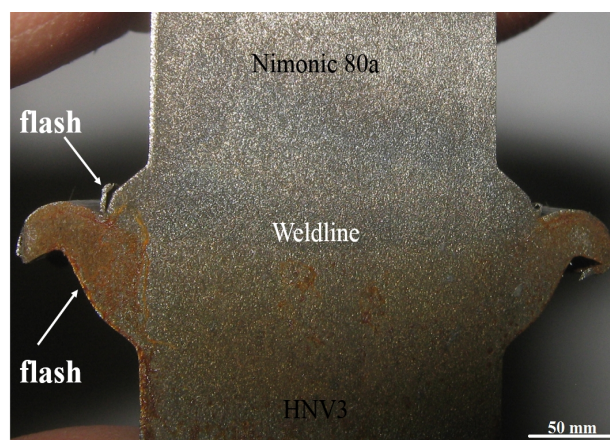
شکل ۱- سطح مقطع اتصال و فلش شکل گرفته در هر دو ناحیه فولادی و سوپراآلیاژی.
