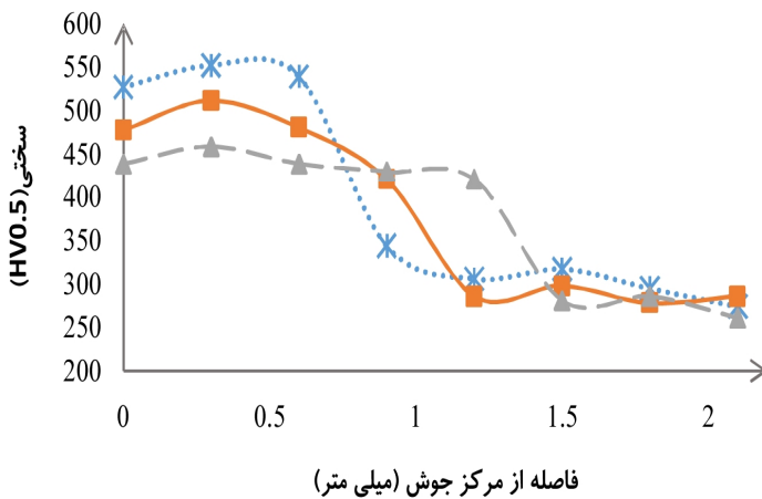
نمودار ۲-پروفایل سختی جوش‌ها
