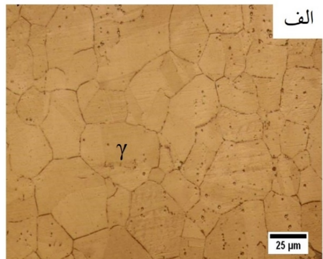
شکل 3- ریز ساختار میکروسکوپ نوری
