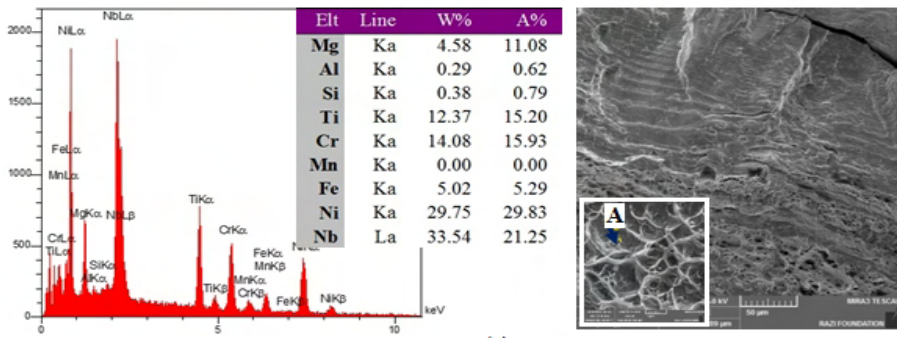
شکل 8- تاثیر ترکیب شیمیایی فلزپرکننده بر سطوح شکست خستگی نمونه‌ها و ترکیب شیمیایی مرکز دیمپلها (نقطه A در شکل‌های مربوطه). (الف) نمونه جوشکاری شده با ER309L، (ب) نمونه جوشکاری شده با ERNiCrMo-3.
