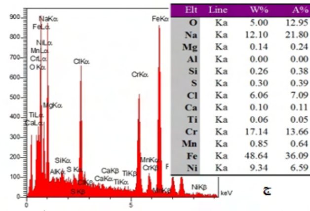
شکل 9- مطالعه سطح شکست خوردگی-خستگی نمونه جوشکاری شده با فلزپرکننده ER309L. (الف) تشکیل حفرات، (ب) تشکیل محصولات غنی از محیط خورنده، (ج) آنالیز EDS از ذرات N. M و N به ترتیب معرف حفرات و محصولات خوردگی در سطح شکست می‌باشد.
