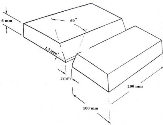
شکل 1- طرح اتصال ورق‌ها برای انجام فرآیند جوشکاری.
