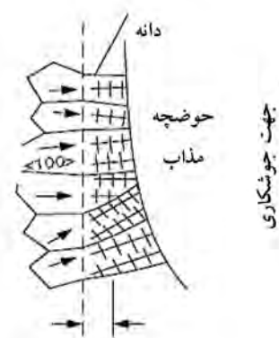
شکل 8- رشد رونشینی در ناحیه خط ذوب [31]
