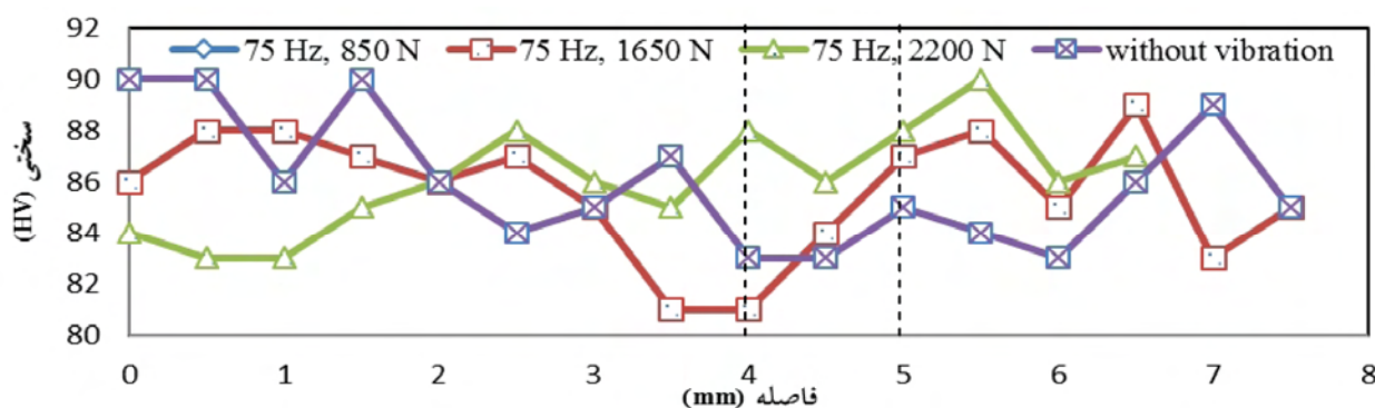
شکل 9- نتایج سختی سنجی نمونه های جوشکاری شده
