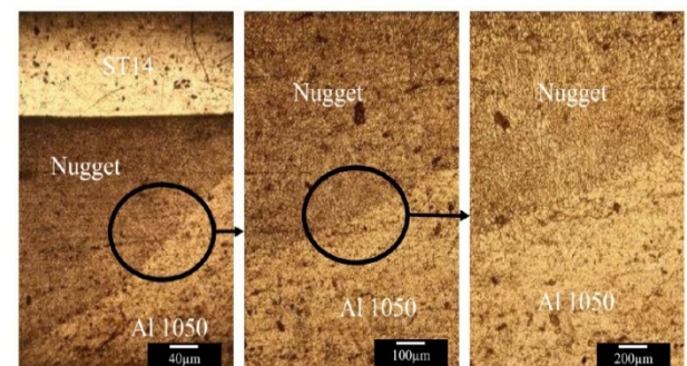
شکل 9- ریزساختار نمونه شماره 8.
