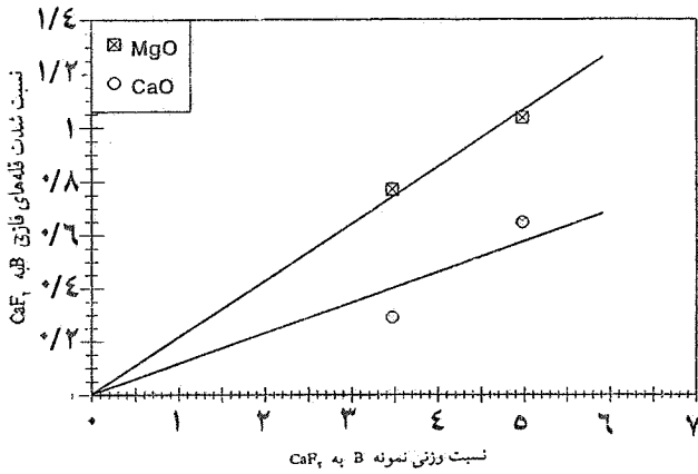
شکل ۴- نسبت شدت قله های فازي نمونه B به CaF ۲ در مقابل نسبت وزنی نمونه B به CaF ۲
