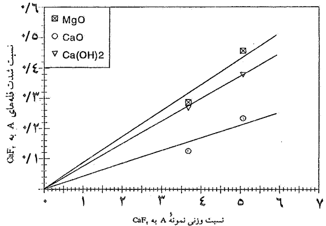
شکل ۳- نسبت شدت قله های فازي نمونه A به CaF ۲ در مقابل نسبت وزنی نمونه A به CaF ۲
