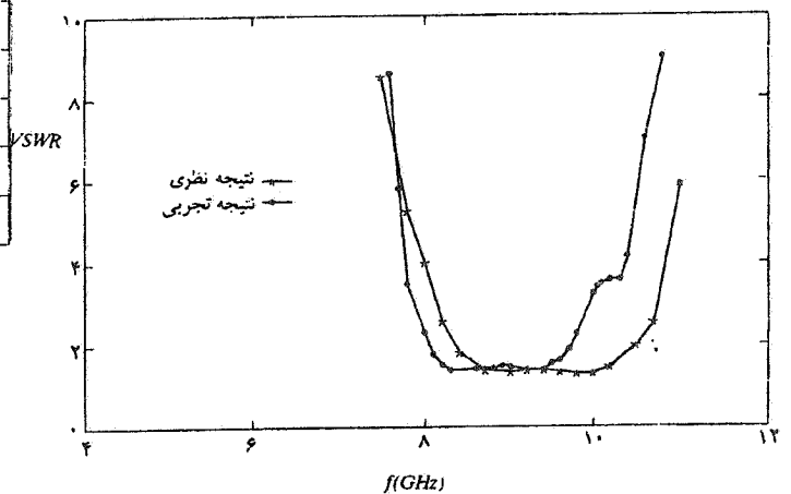
شکل ۷- نتیجه تجربی و نظری برای VSWR آنتن مثال (۴)، w_a=0/3\text{cm} ، d_a=0/75\text{cm} ، b=1/1\text{cm} ، a=0/7\text{cm} ، d_1=0/317\text{cm} ، \epsilon_{rf}=6/15 ، w_f=0/09\text{cm} ، d_s=0/11\text{cm} ، d_f=0/0614\text{cm}
