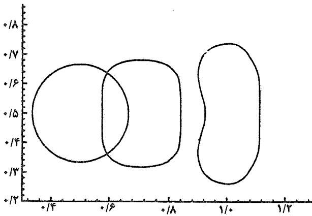
شکل ۱۰- تغییر شکل قطره در We=4 Re_l=200 و Re_g=1
