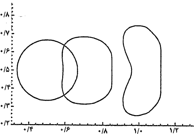
شکل ۱۱- تغییر شکل قطره در We=4 Re_l=200 و Re_g=5
