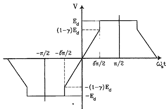
شکل ۴- نتایج رایانه‌ای مربوط به شبیه‌سازی اینورتر T p PWM با m_a = 0.8 ، m_f = 15 ، \sigma = 0.33 و \gamma = 0.38
