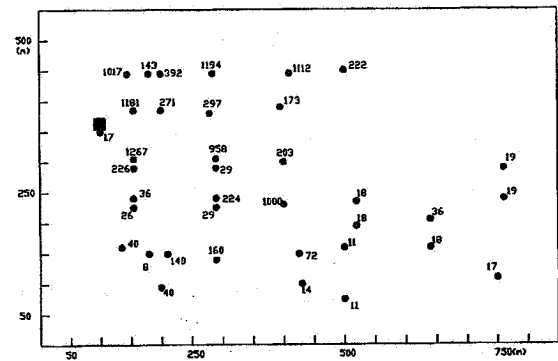
شکل ۱- مراکز بار و محل تغذیه اصلی در یک کارخانه شیمیایی در
