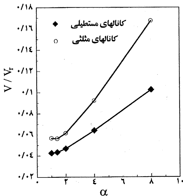
شکل ۴- تغییرات نسبت حجم مبدل با کانالهای مستطیلی و مثلثی به حجم مبدل سطح مینا بر حسب α در حالت FG-1a, FG-1-b
