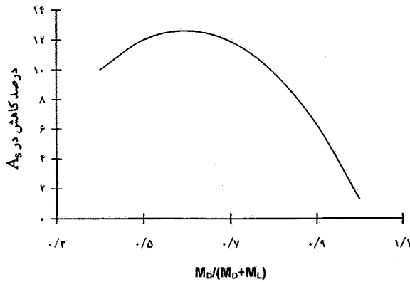
شکل ۴- درصد کاهش مصرف فولاد در طراحی به روش تمام احتمالاتی در مقایسه با روش آیین نامه‌ای
