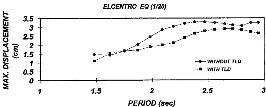
شکل ۱۴- تغییرات پاسخ حداکثر سازه‌ها
