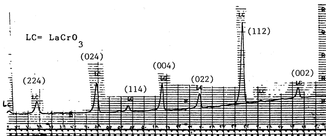
شکل ۴- الگوی پراش پرتو X ترکیب لانتانیوم کرومیت کلوغه شده در دمای 1300^\circ\text{C}
