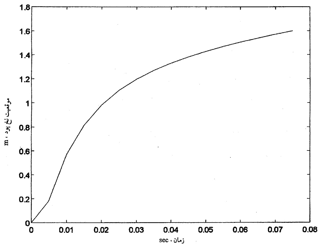
شکل ۲- نمودار موقعیت نوک نخ پود برحسب زمان به هنگام پودگذاری
