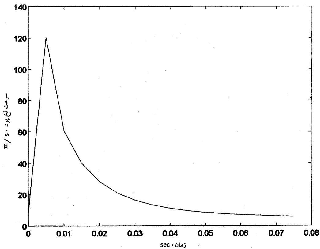
شکل ۳- نمودار سرعت نوک نخ پود برحسب زمان به هنگام پودگذاری
