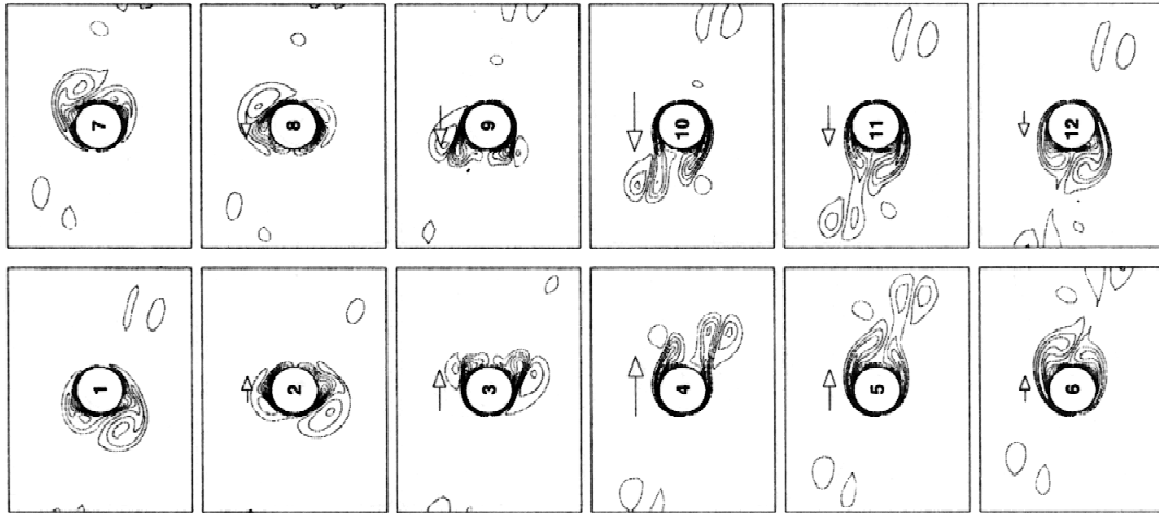
شکل ۶- از راست به چپ به ترتیب خطوط ورتیسیتی و خطوط جریان برای حالت‌های استوانه نوسانی و جریان نوسانی به ازای \beta = 35 , KC = 8.0
