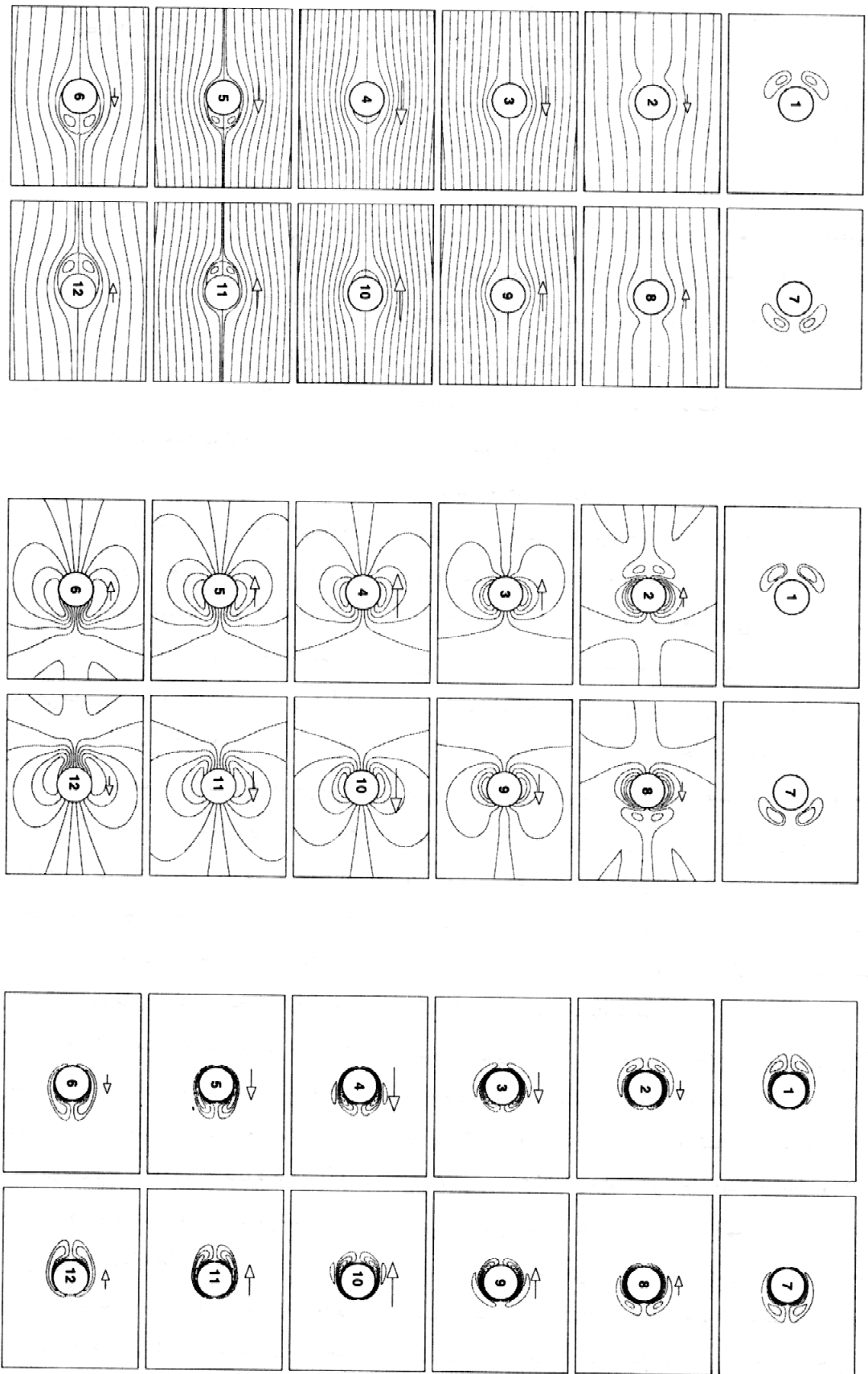
شکل ۳- از راست به چپ به ترتیب خطوط جریان و خطوط استوانه نوسانی و جریان نوسانی به ازای \beta = 3.5 , KC = 4.0
