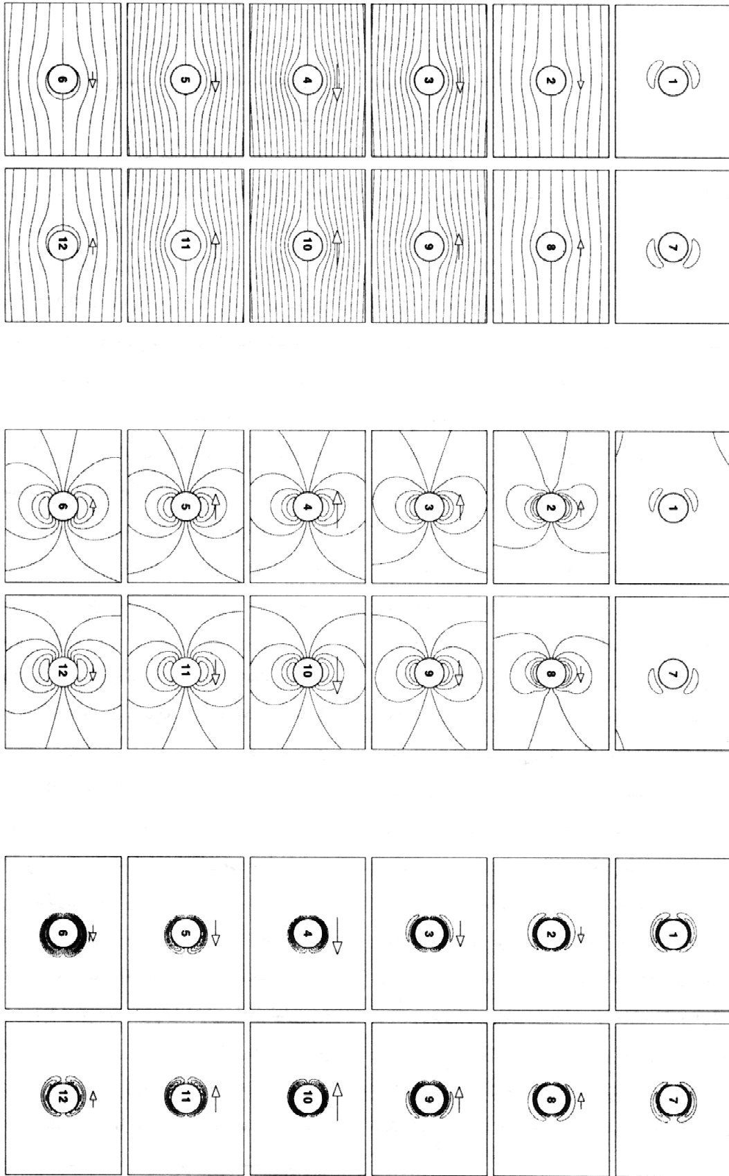
شکل ۱- از ازا- تا ازا-۱۲: خطوط پتانسیل، خطوط جریان و استریم‌لاین‌های استوانه نوسانی و جریان نوسانی به ازای \beta = 35 ، KC = 1.0
