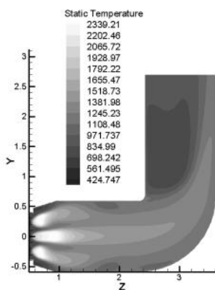
شکل ۱۳- توزیع دما در محفظه زانویی
