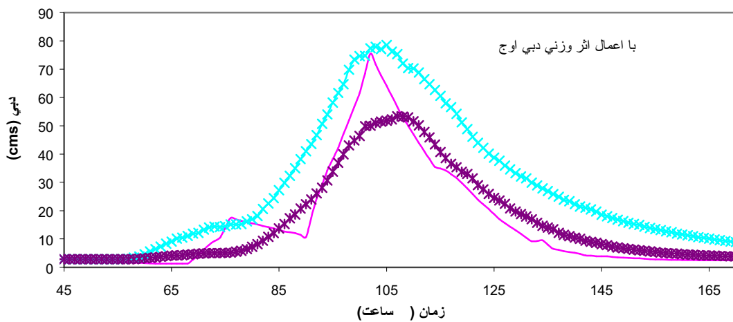
شکل ۱۲- محدوده پیش‌بینی با اثر یکسان و اثر وزنی دبی هیدروگراف سیلاب مورخ ۱۸ آذر ۵۷
