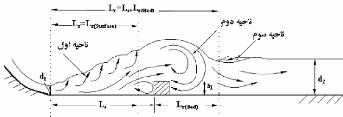
شکل ۱۲- انواع گرداب تشکیل شده در تشکیل پرش با وجود یک دیواره
