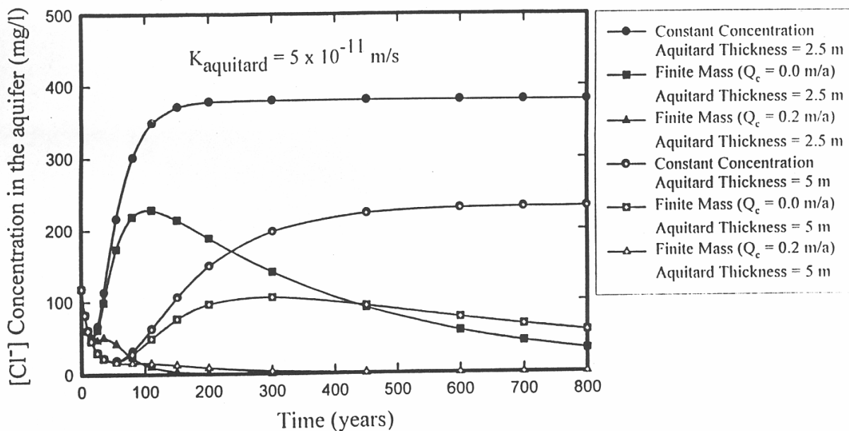
شکل ۹ - تغییرات غلظت یون کلر (Cl) در سفره آبدار نسبت به زمان در مدفن زباله با زهکش سفره ای (گزینه سوم) در حالت (۱) تاثیر غلظت ثابت نسبت به غلظت یا جرم محدود در کف مدفن، (۲) تاثیر ضخامت لایه زمین طبیعی، و (۳) تاثیر میزان زهکشی شیرابه در کف مدفن. K_{aquitard} = 5 \times 10^{-11} (m/s)
