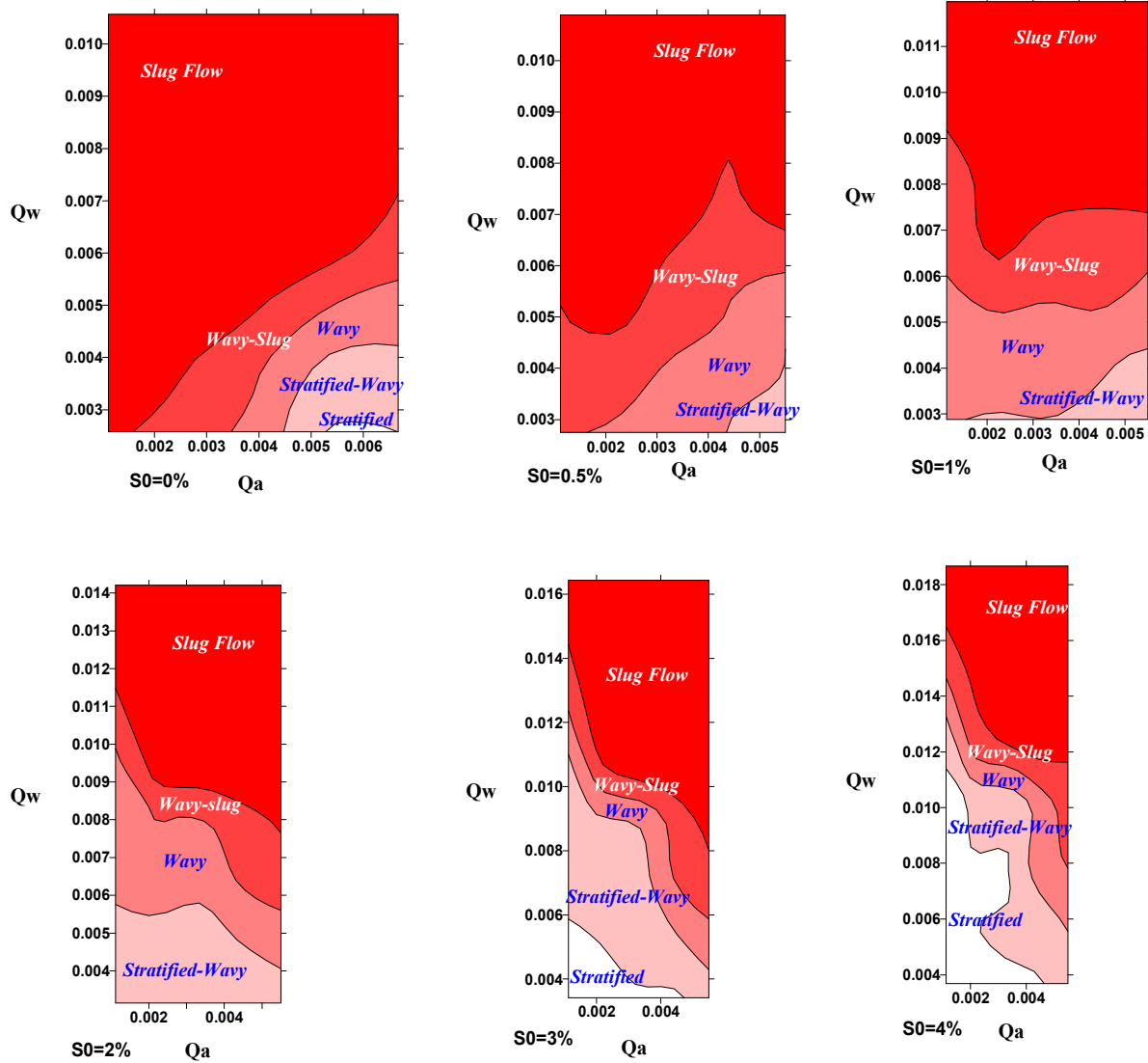
شکل ۵- نقشه الگوهای جریان محتمل در تونلها و مجاری با قطر زیاد برای شیبه‌های مختلف (دییها بر حسب متر مکعب بر ثانیه هستند).
