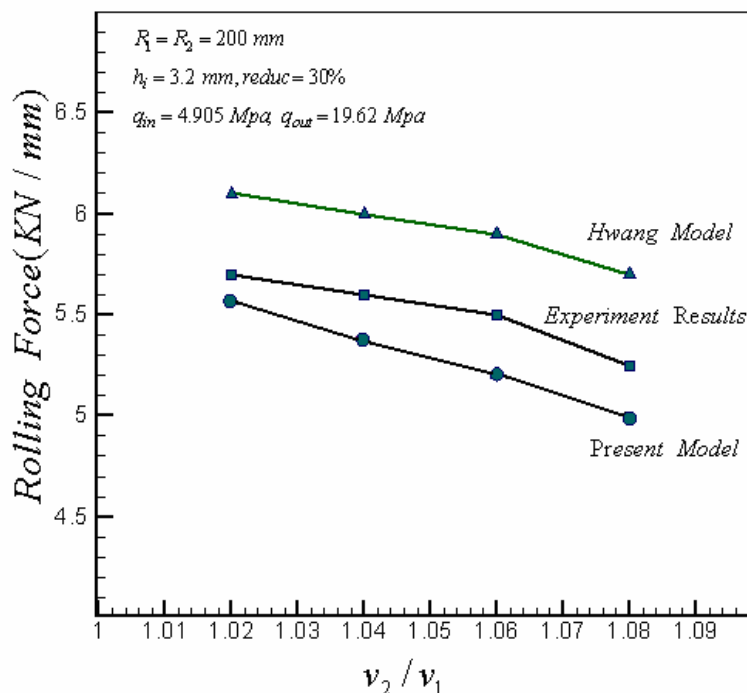
نمودار ۱۶- مقایسه نیروی نورد به دست آمده از مدل حاضر با مدل هوانگ [۱۹] و نتایج تجربی [۲۴]
