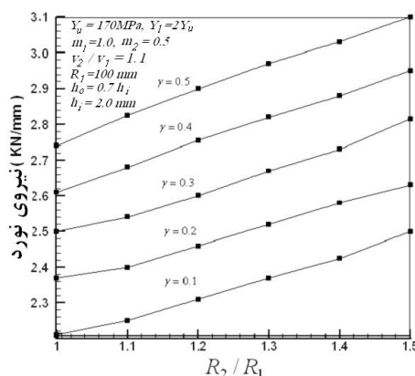
شکل ۹- تغییرات نیروی نورد بر اساس نسبت‌های مختلف شعاع‌های دو غلتک و برای نسبت‌های مختلف از ضخامت‌های دو لایه ورق
