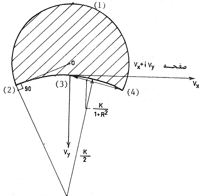
شکل ۶- هودوگراف سرعت
