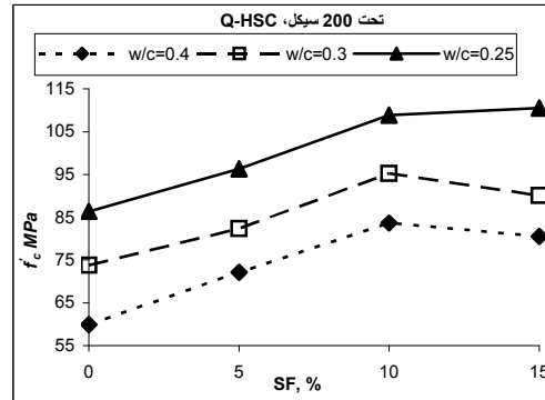
شکل ۱۱- مقاومت فشاری بتن با درشت دانه کوارتزی در مقابل درصدهای میکروسیلیس بعد از ۲۰۰ سیکل
