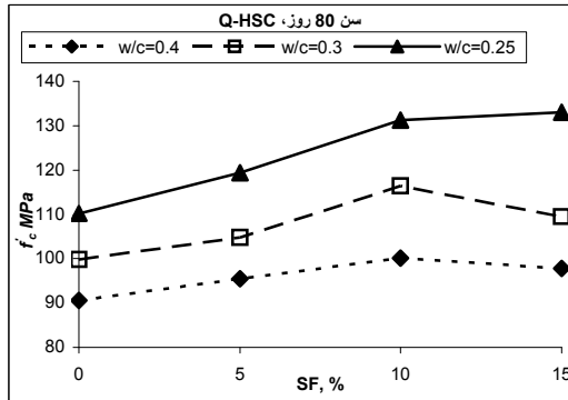
شکل ۱۲- مقاومت فشاری بتن شاهد با درشت دانه کوارتزی در مقابل درصدهای میکروسیلیس بعد از ۸۰ روز
