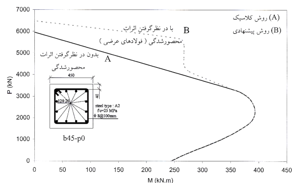
شکل ۵ - نمودار اندرکنش بار محوری - لنگر خمشی نمونه b45-p0
