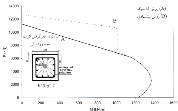
شکل ۶ - نمودار اندرکنش بار محوری - لنگر خمشی نمونه b45-p1.2
