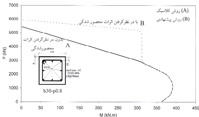
شکل ۴ - نمودار اندرکنش بار محوری - لنگر خمشی نمونه b30-p0.8
