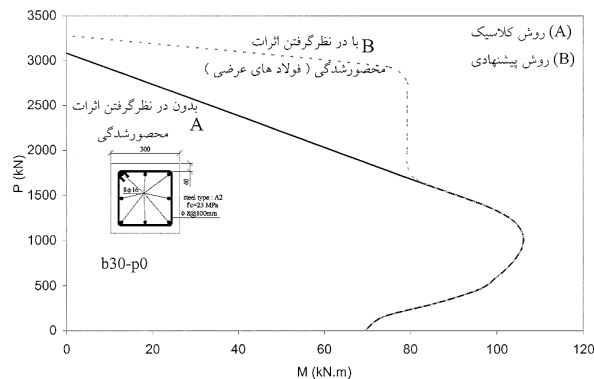
شکل ۳ - نمودار اندرکنش بار محوری - لنگر خمشی نمونه b30-p0
