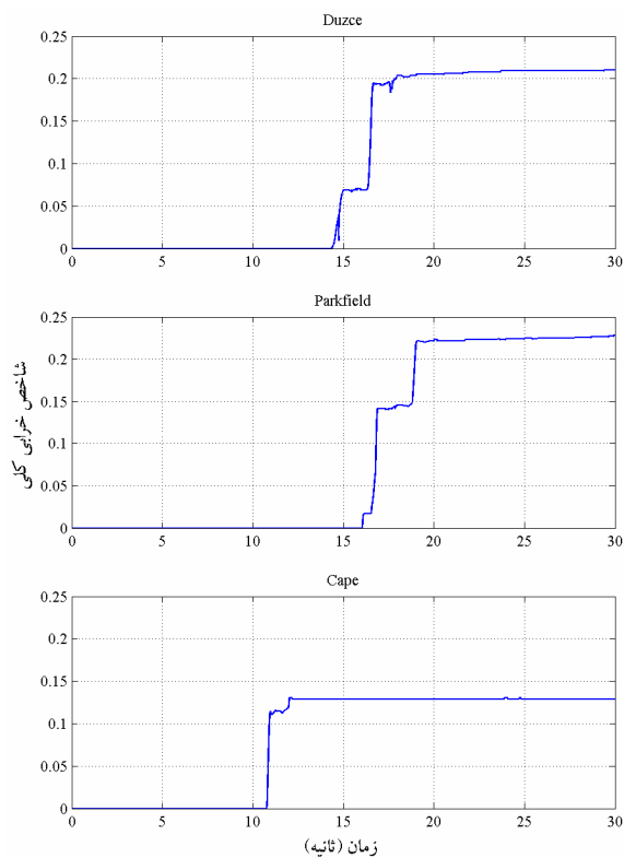
شکل ۱۷- تاریخچه شاخص خرابی کلی سازه برای دوره بازگشت ۱۰۰۰ ساله
