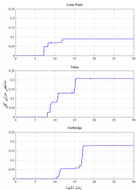
شکل ۱۷- تاریخچه شاخص خرابی کلی سازه برای دوره بازگشت ۱۰۰۰ ساله
