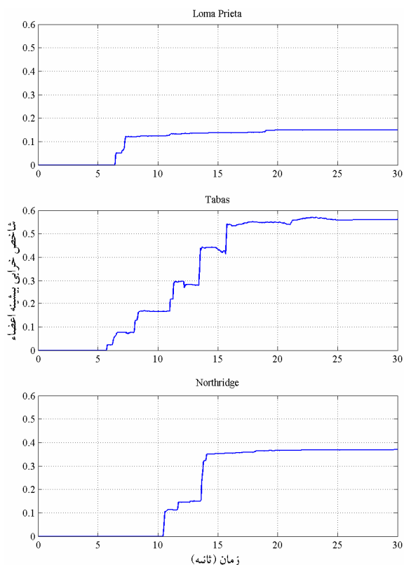
شکل ۱۸- تاریخچه شاخص خرابی بیشینه اعضا برای دوره بازگشت ۲۵۰۰ ساله
