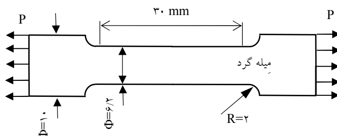
شکل ۷- هندسه نمونه کششی، مطابق استاندارد ASTM E8-04
