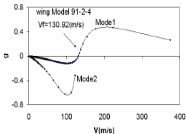
شکل ۵ - سرعت بر حسب g برای بال سری ۹۱-۲-۴ آزمایش تجربی [۲۲] و روش حاضر
