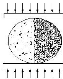
شکل ۱- آزمایش دو نیم شدگی نمونه استوانه‌ای
