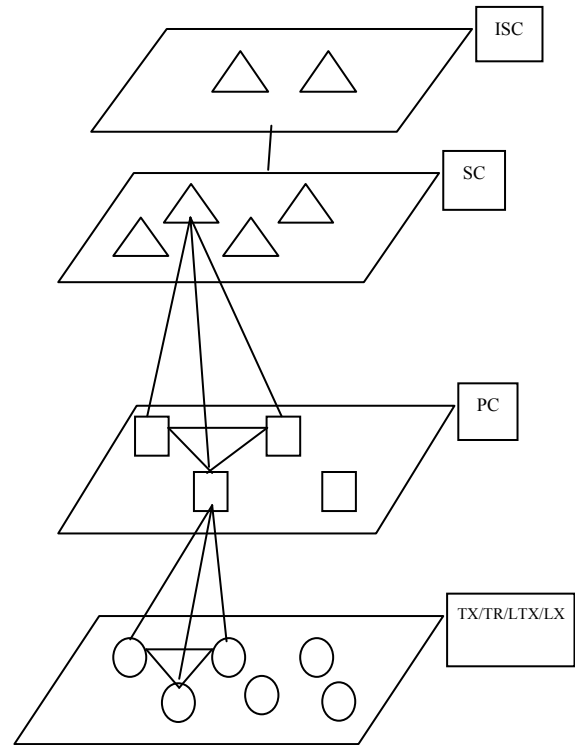
شکل ۱- ساختار سلسله مراتبی شبکه تلفنی ثابت کشور
