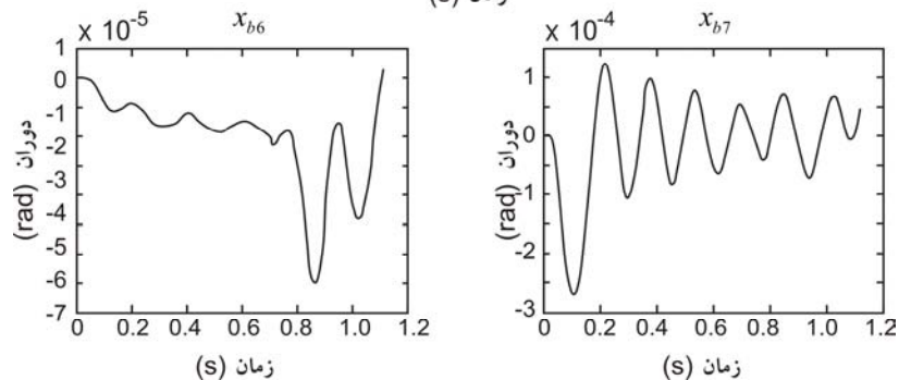
شکل ۱۲- انتقال قائم (پرش) و دوران قاب بوژی برای یک مدل بوژی کامل عبوری از تکه مرکزی
