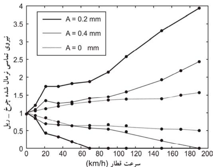
شکل ۱۳- حداکثر و حداقل نیروهای تماسی نرمال شده ریل - چرخ بر تکه مرکزی (نیروی تماسی نرمال شده استاتیکی) برحسب سرعت وسیله نقلیه برای سه حالت ناهمواری متفاوت (۰، ۲، ۴ و ۰ میلی‌متر) به کار رفته در مدل نیم بوژی
