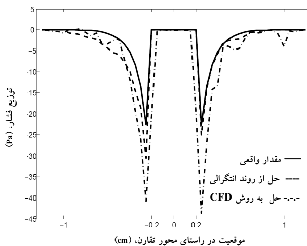
شکل ۱۰- توزیع فشار در محور تقارن مدل جریان کوئنت از محاسبات ریاضی معادله (۳۲) (خط پر) با استفاده از حل انتگرالی حاضر (خط چین) و از روشهای متداول دیفرانسیلی (خط نقطه) وقتی داده های اولیه سرعت با همهمه ترکیب شده اند
