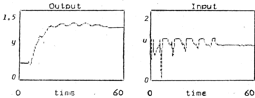
شکل ۲۰- پاسخ نسبت به تغییر پله‌ای در y_r با کنترل کننده پس خور معادل IMC با وجود محدودیت در ورودی بدون آنتی وا ایند آپ (مثال ۲)
