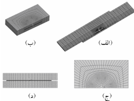
شکل ۶- مدل و زیرمدل اجزای محدود شبکه بندی شده اتصال در نماهای مختلف
