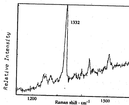
شکل ۴ - پوشش تشکیل شده در نسبت اکسیژن به استیلن برابر ۹/۰
