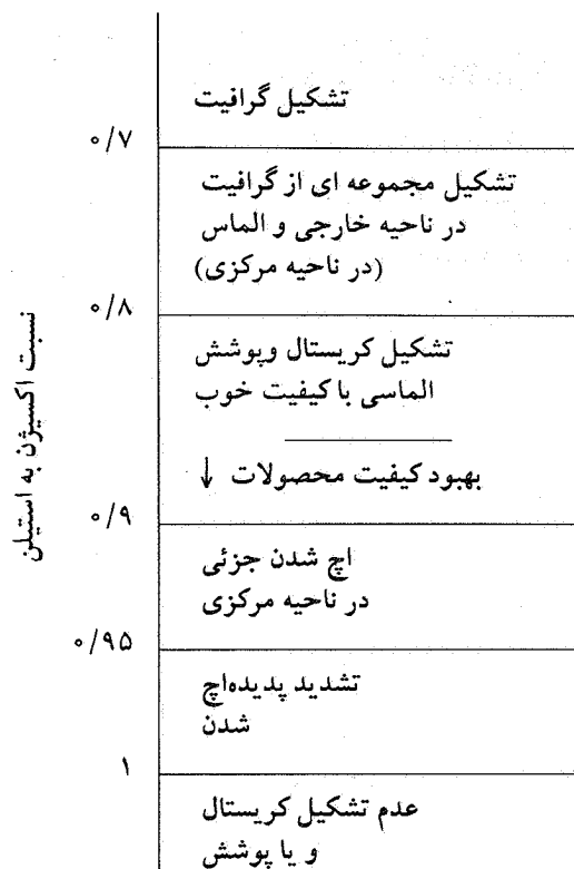
شکل ۶ - اثر نسبت گاز اکسیژن به استیلن در تشکیل و کیفیت پوششهای الماسی
