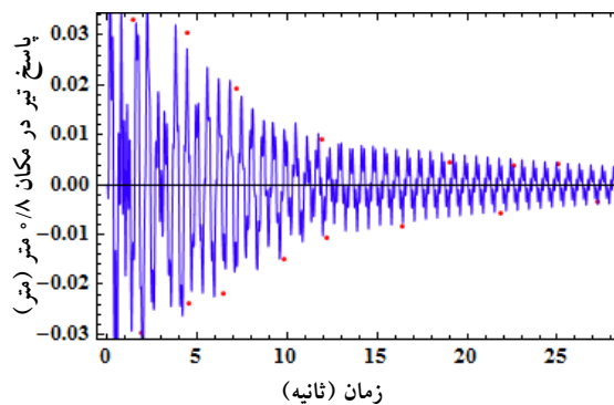
شکل ۳- (رنگی در نسخه الکترونیکی) مقایسه پاسخ تیر در مکان ۰/۸ متر؛ خطوط پیوسته مربوط به مدل حاضر، و منحنی نقطه چین مربوط به مرجع [۱۹]
