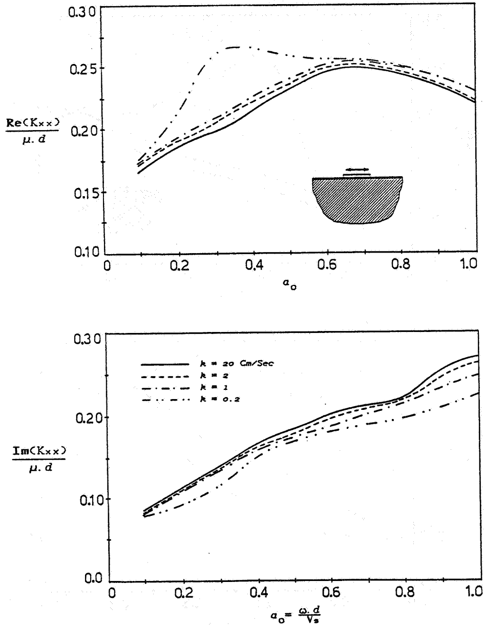
شکل ۱۳ - مقایسه محیط متخلخل اشباع با نفوذ پذیری بالا و محیط خشک تک فاز در تعیین سختی چرخشی دینامیکی پی صلب
