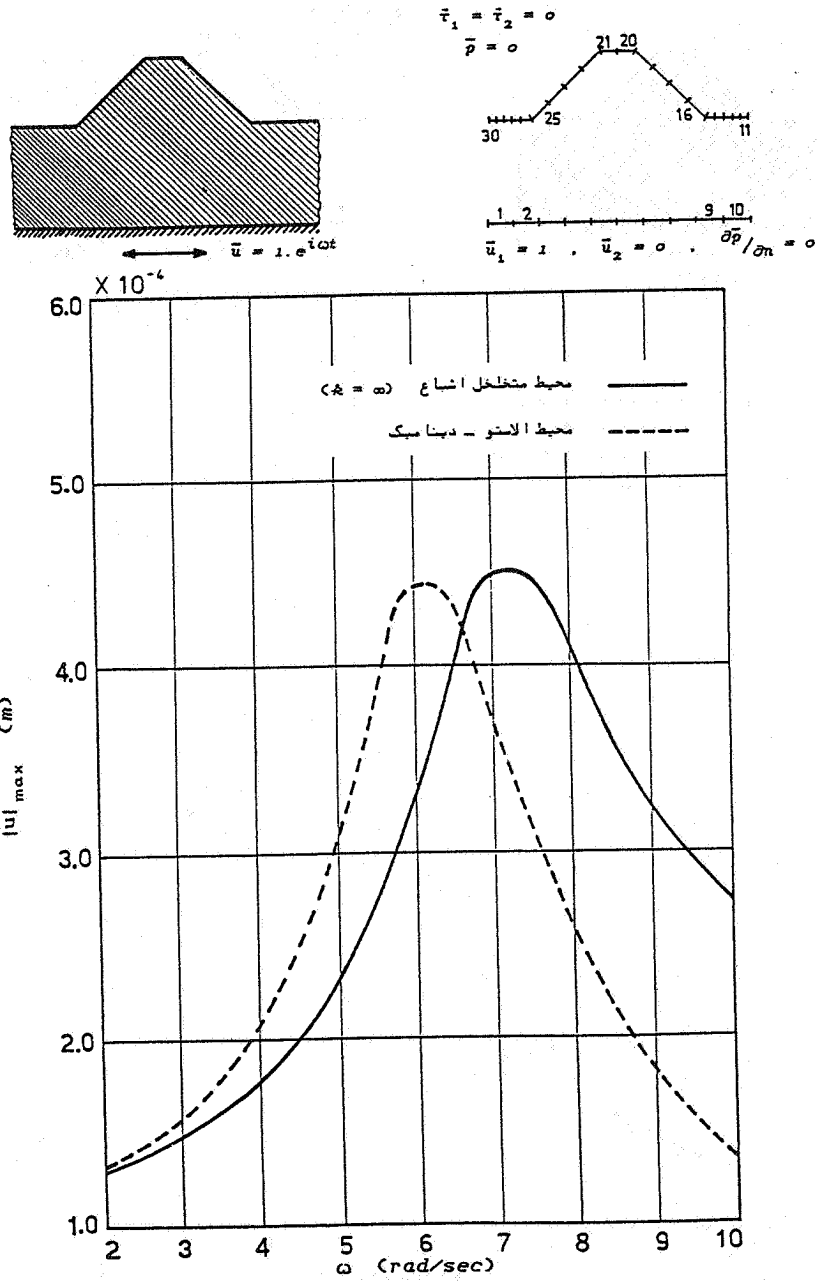
شکل ۵ - مقایسه محیط متخلخل اشباع (k = \infty) با یک محیط الاستودینامیک در تغییر مکان تاج سد
