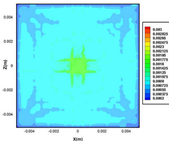
شکل ۶- توزیع کسر حجمی نانوذرات اکسید مس در انتهای کانال (y = 5° cm) در کسر حجمی متوسط \phi = 0/1\% و
